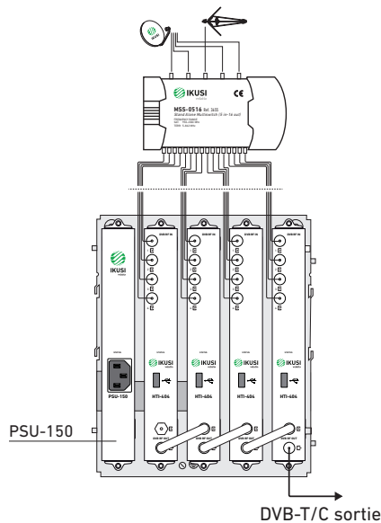
Exemple d'installation contenant 4 transmodulateurs HTI + 1 source d'alimentation PSU-150.
