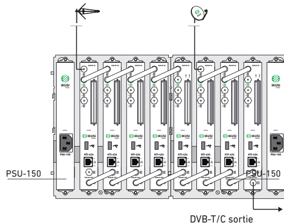
Exemple d'installation contenant 8 transmodulateurs HTI + 2 sources d'alimentation PSU-150, montés sur 2 platines BACK-500 connectées par le pont USB.
